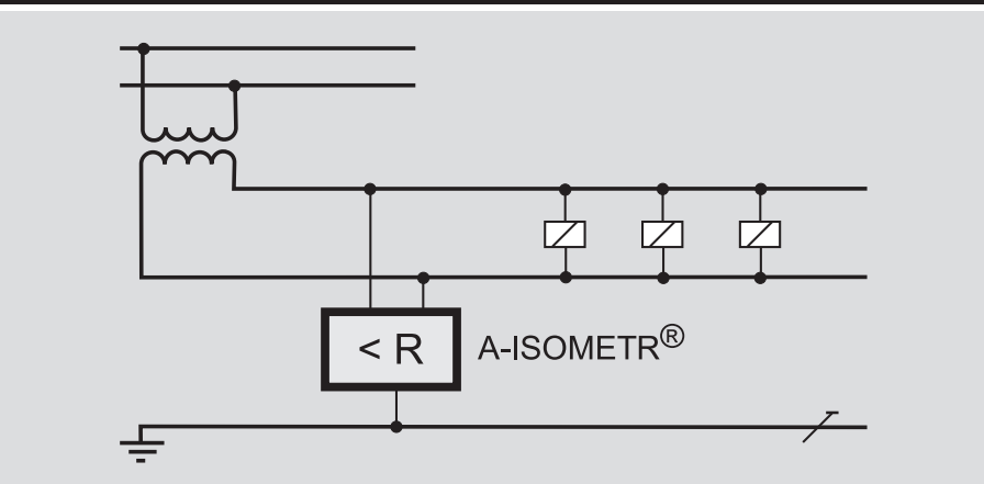
AC (střídavé) řídicí obvody
