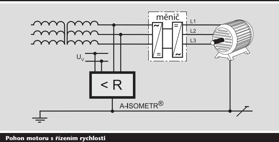
Pohon motoru s řízením rychlosti
