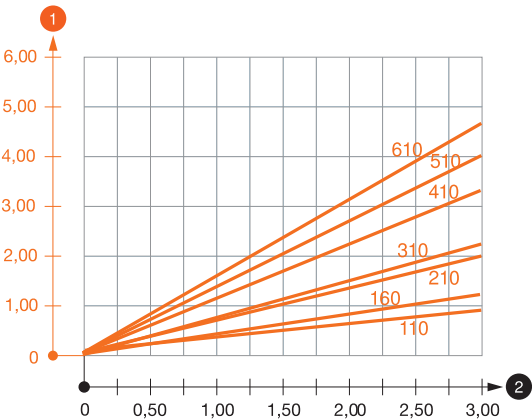
Zatěžovací diagram výložníku typu AS 30
