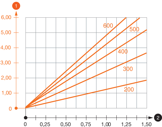
Zatěžovací diagram výložníku typu AS 15
