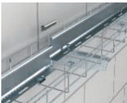
Šroubové upevnění přepážky
