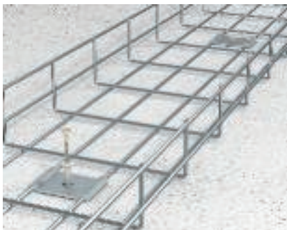
Přímé upevnění na podlahu
