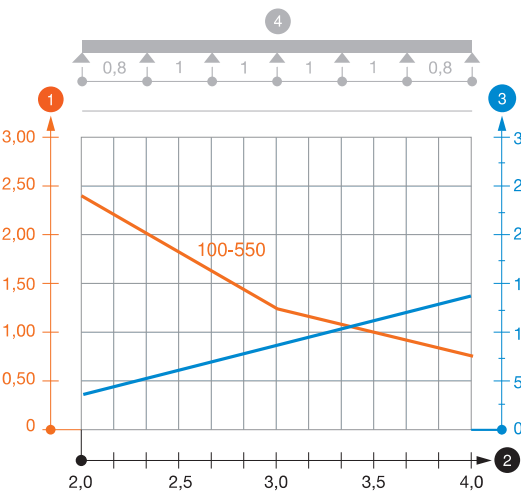
Zatěžovací diagram kabelového žlabu typu SKSU 110
