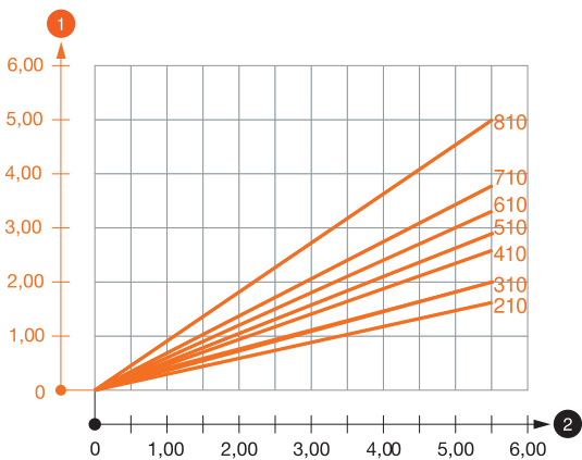
Zatěžovací diagram výložníku typu AS 55
