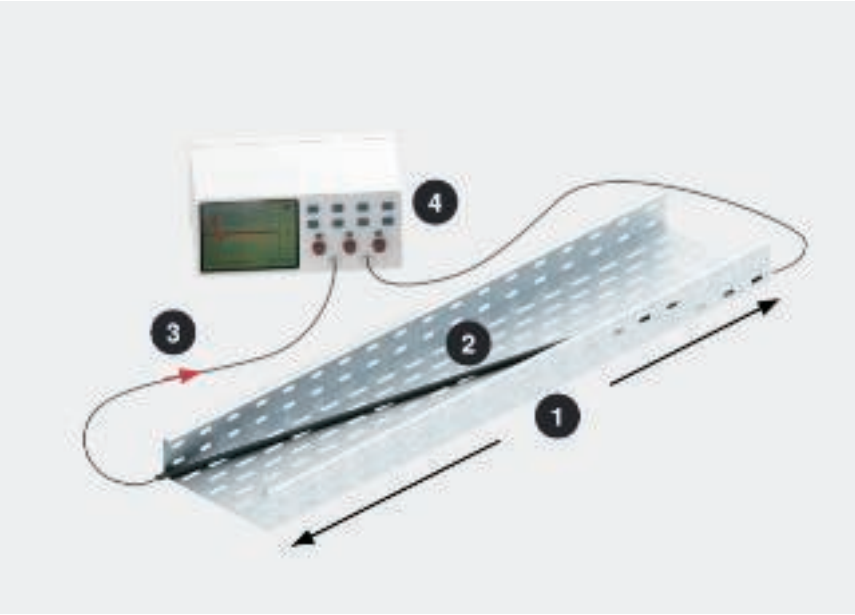
Pokusný model k měření přenosové impedance: 1 = délka L, 2 = U, 3 = I, 4 = zdroj impulsů 8/20
