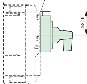
NZM3-XDV NZM3-XDVR
